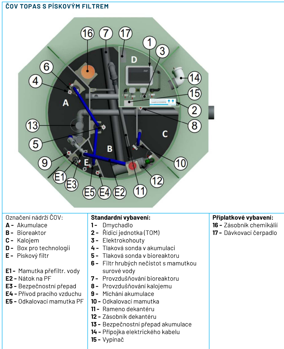
Obrázek 1: Půdorysné schéma TOPAS S
